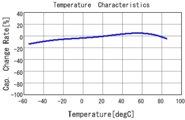
■ GRM31CR60J227ME11 C-Temp. capchange, DCO. 0V, ACO. 1Vrm
