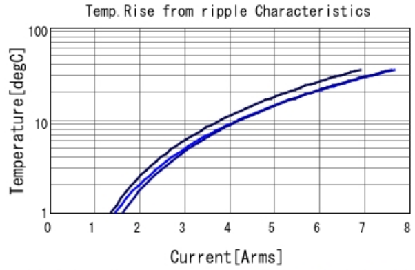
GRM31CR60J227ME11 Temp. rise ■ 50kHz ■ 200kHz ■ 400kHz
