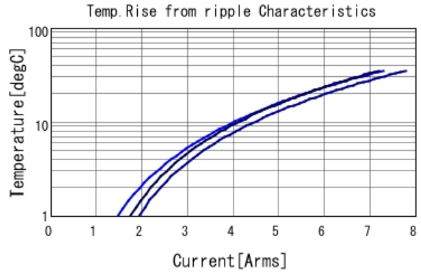
GRM32EC70G107ME15 Temp. rise ■ 50kHz ■ 200kHz ■ 400kHz
