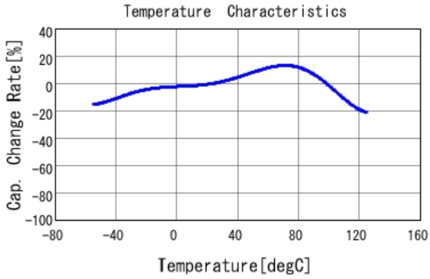
■ GRM32EC70G107ME15 C-Temp. capchange, DCO. 0V, ACO. 18Vr
