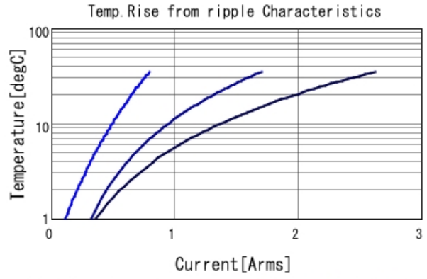
GRM55DR72E334KW01 Temp. rise ■ 30kHz ■ 100kHz ■ 300kHz
