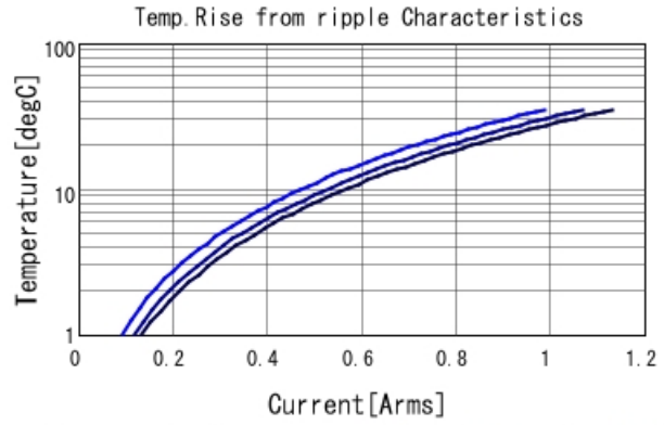
■ GRT033R61E104KE01 Temp. rise ■ 400kHz ■ 800kHz ■ 1MHz
