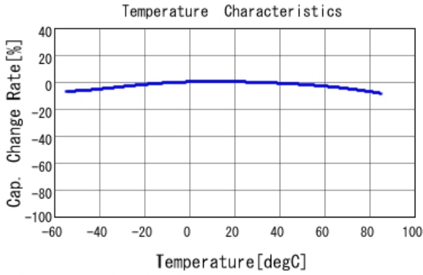
■ GRT033R61E104KE01 C-Temp. capchange, DCO. 0V, ACO. 5Vrm
