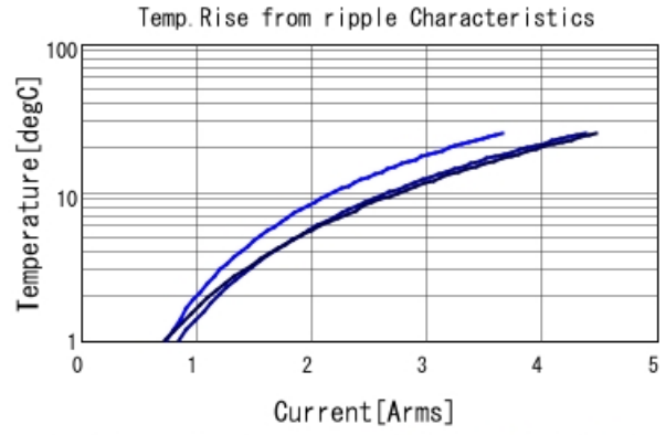
KCM55QR72A685KH01 Temp. rise ■ 50kHz ■ 100kHz ■ 300kHz
