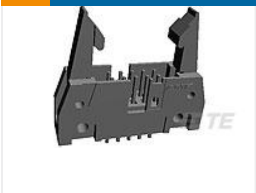
TE Part #5499910-1 A/L UNIV HDR 10P VERT SHT LAT
