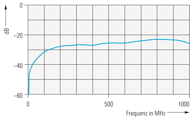
Typische Kennlinie im Frequenzbereich 30 MHz bis 1 GHz
