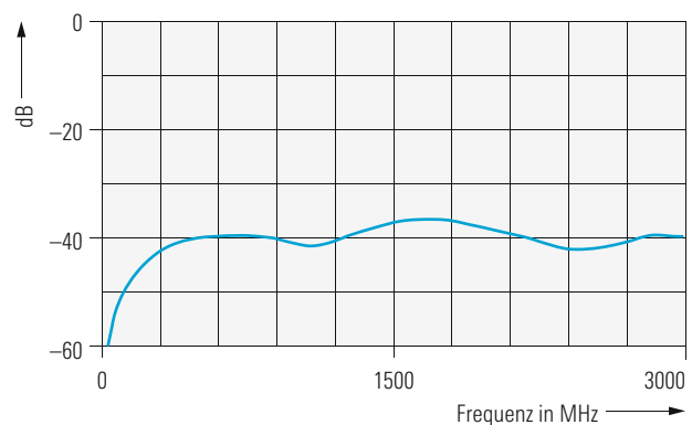
Typische Kennlinie im Frequenzbereich 30 MHz bis 3 GHz
