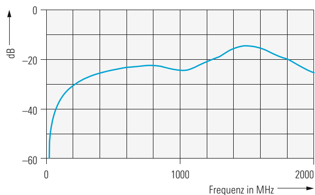
Typische Kennlinie im Frequenzbereich 30 MHz bis 2 GHz
