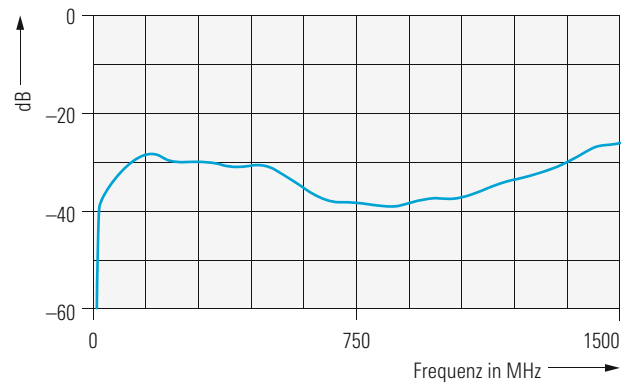
Typische Kennlinie im Frequenzbereich 30 MHz bis 1,5 GHz
