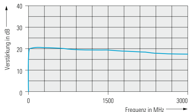
Typischer Frequenzgang
