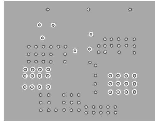
Inner Layer 1
