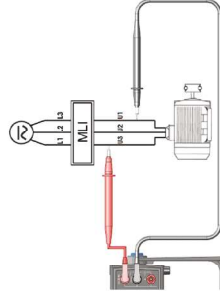
Exemple : mesure de tension sur un variateur
