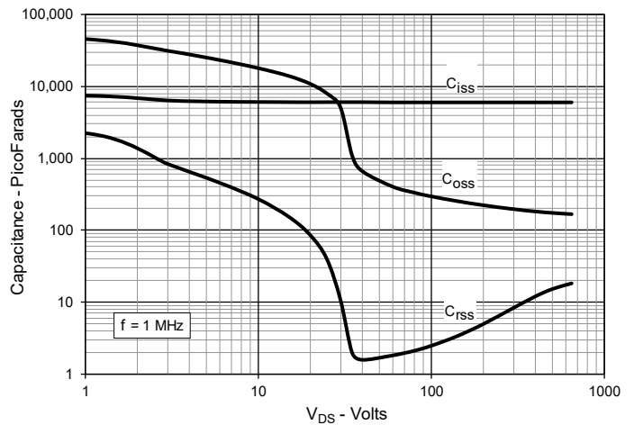
Fig. 12. Capacitance
