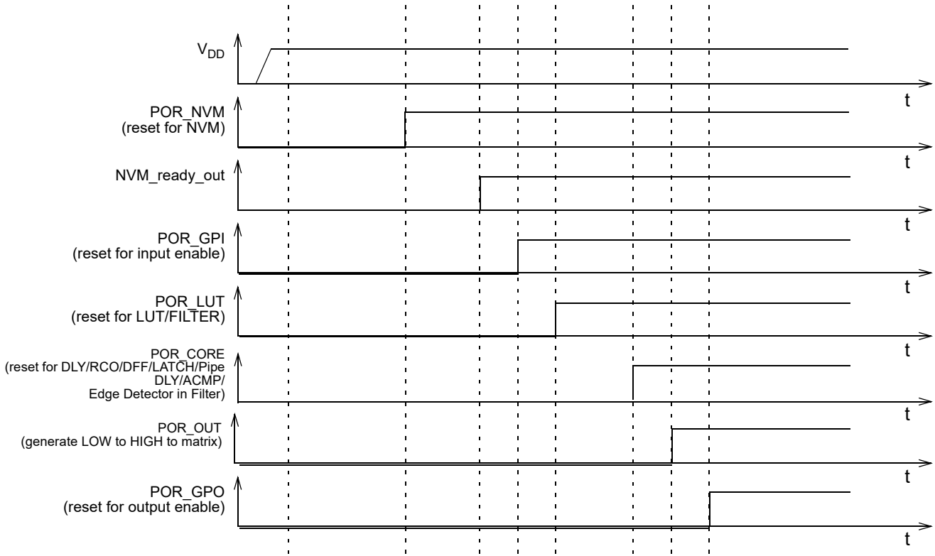
Figure 134. POR Sequence
