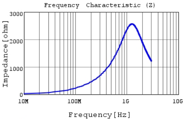
LQW18CNR39J0H |Z|
