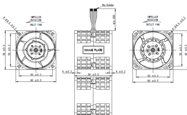
(Outline)
