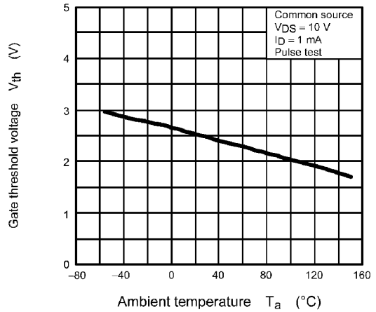
Fig. 8.10 V_{th} - T_a
