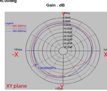
Theta=90.00deg
