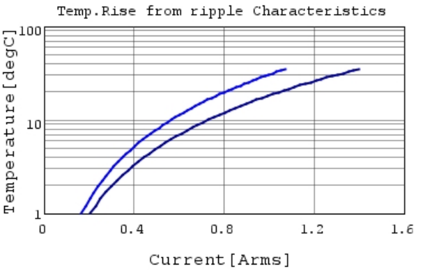
GRM155R71H104KE14 Temp.rise 500kHz
