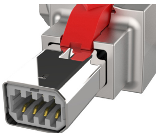
Type I (D) Mating Interface
