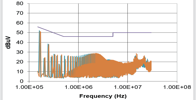
MGJ2D121805BSC (Average)
