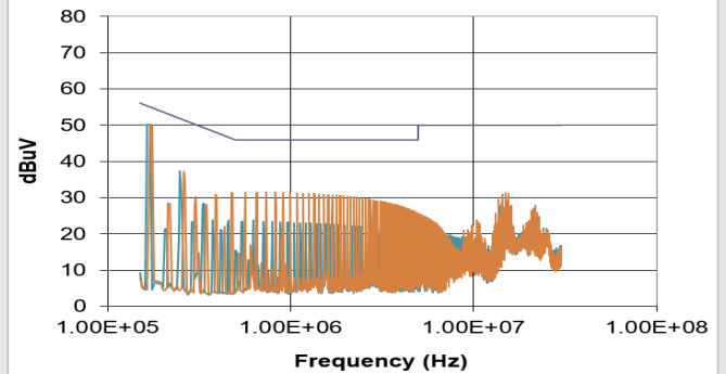
MGJ2D121802BSC (Average)
