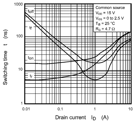
Fig. 7.1.10 t - I_D
