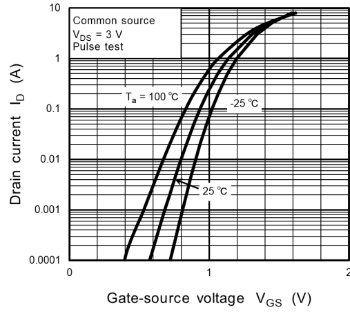
Fig. 7.1.2 I_D - V_{GS}
