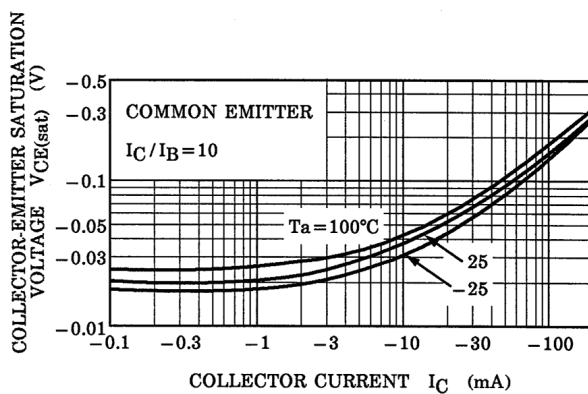
Fig. 8.3 V_{CE(sat)} - I_C
