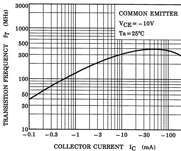
Fig. 8.5 f_T - I_C
