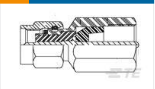
TE Part #1-1337562-0 FME Str Plg-BNCP Adp Nickel Pltd
