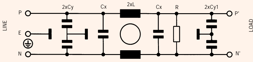
FN 9676 (16A)
