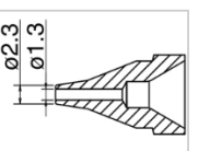
N61-06 Nozzle S type Size Φ1.3
