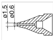
N61-01 Nozzle SS type Size Φ0.6
