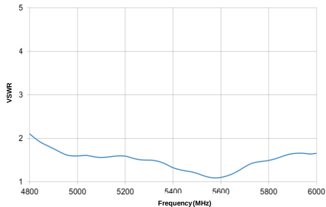
5 GHz VSWR
