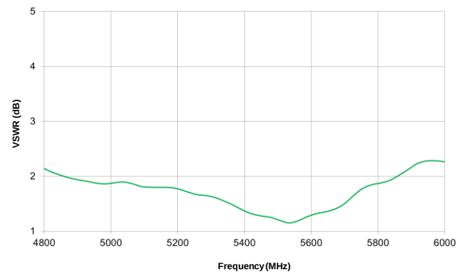
5 GHz VSWR
