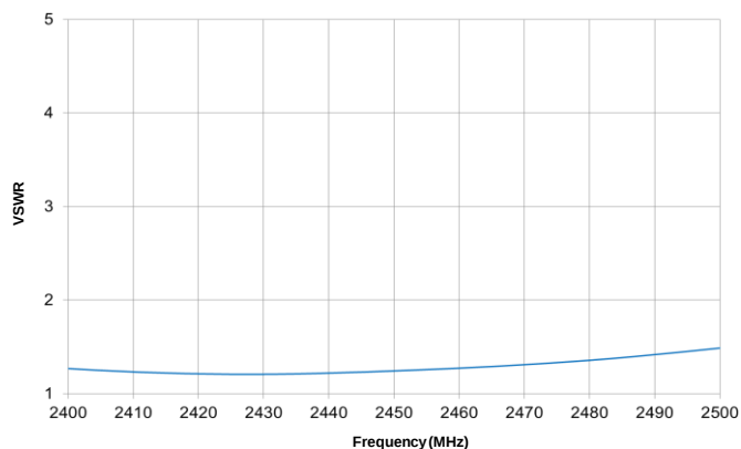
2.4 GHz VSWR
