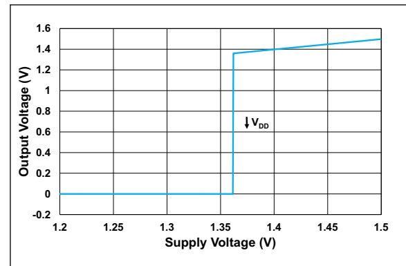
FIGURE 4-6: POR Falling.
