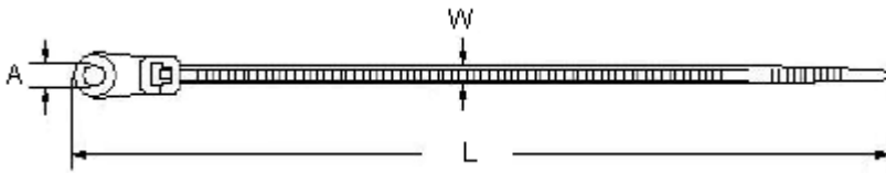
Dimensions : Millimetres
