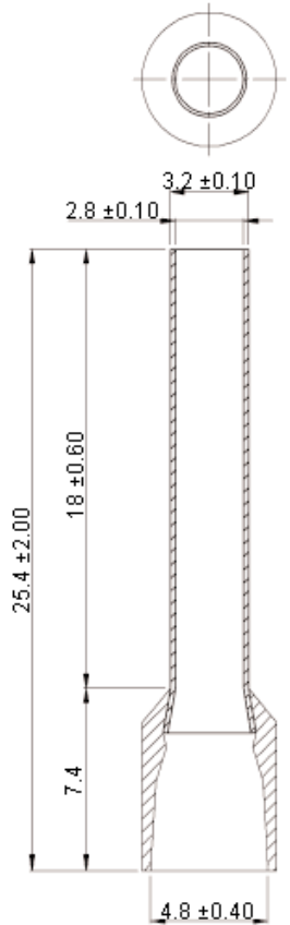
Dimensions : Millimetres
