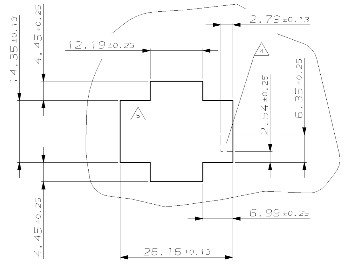
Montageausschnitt / PANEL CUT OUT Bestückungsseite / LOADING SIDE M 2:1 / SCALE 2:1
