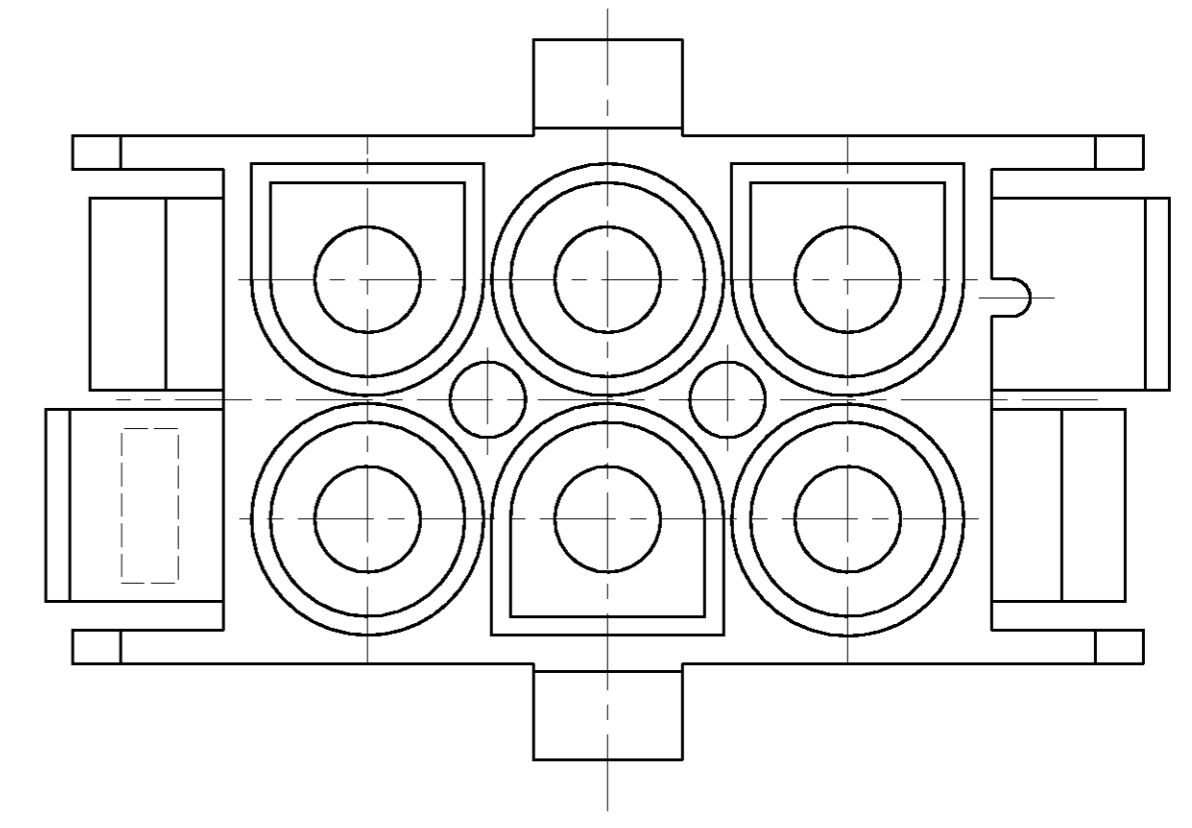
Montageausschnitt / PANEL CUT OUT Bestückungsseite / LOADING SIDE M 2:1 / SCALE 2:1
