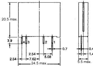
G3MB-202P□□□-4
