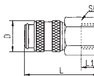
Innengewinde
