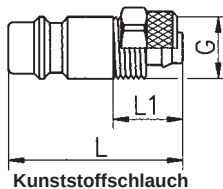
Kunststoffschlauch
