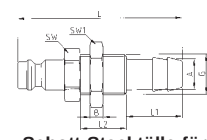
Schott-Stecktülle für Schlauchanschluss
