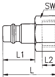
Innengewinde
