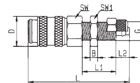
Schottverschraubung für Kunststoffschlauch
