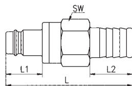
Schlauchanschluß
