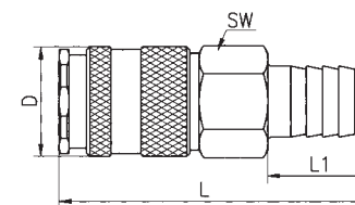
Schlauchanschluß
