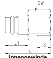
Innengewinde
