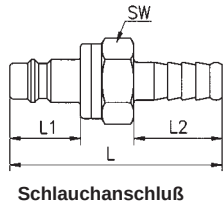
Schlauchanschluß
