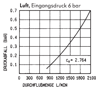
Durchflußdiagramm Einhandkupplung DN 7,8 = 48 mm 2
