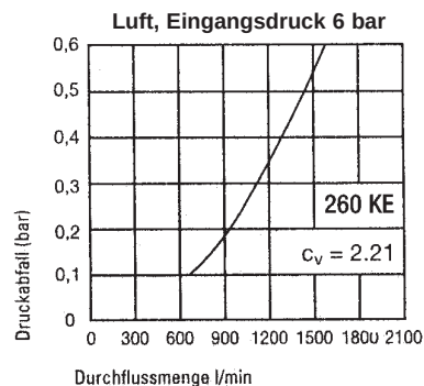
Durchflußdiagramm Einhandkupplung DN 7,4 = 43 mm 2
