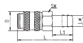
Schlauchanschluß
