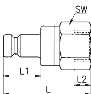
Innengewinde
