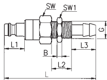
Schottverschraubung für Schlauchanschluß
