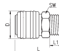
Außengewinde
