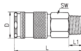
Außengewinde
