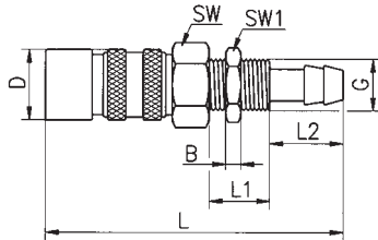
Schottverschraubung mit Schlauchanschlu 
