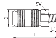
Außengewinde
