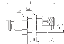
Schott-Stecktülle für Kunststoffschlauch
