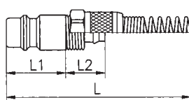
Knickschutzfeder
