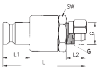
Schlauchanschluß
