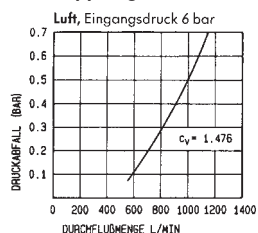
Durchflußdiagramm Einhandkupplungen DN 7,2 = 48 mm 2
