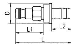
Schlauchanschluß
