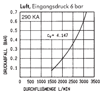
Durchflußdiagramm Einhandkupplung DN 13 = 130 mm 2
