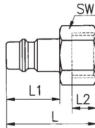
Innengewinde
