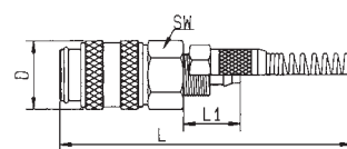
Knickschutzfeder
