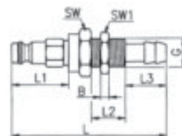
Schottverschraubung für Schlauchanschluß
