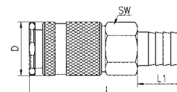
Schlauchanschluß
