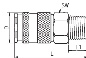
Außengewinde
