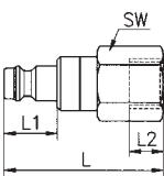
Innengewinde
