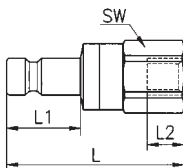
Innengewinde
