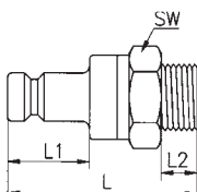
Außengewinde
