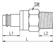
Außengewinde
