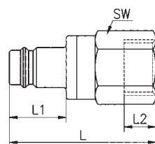
Innengewinde
