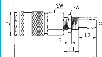
Schottverschraubung für Schlauchanschluß
