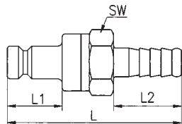
Schlauchanschluß
