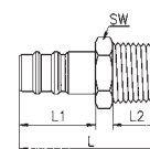
Außengewinde
