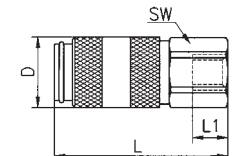
Innengewinde
