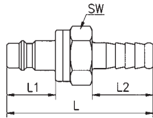
Schlauchanschluß
