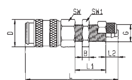
Schottverschraubung für Kunststoffschlauch
