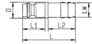
Schlauchanschluß
