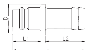
Schlauchanschluß
