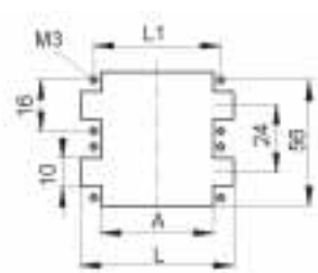
Montageausschnitt Panel cut-out Découpe de montage
