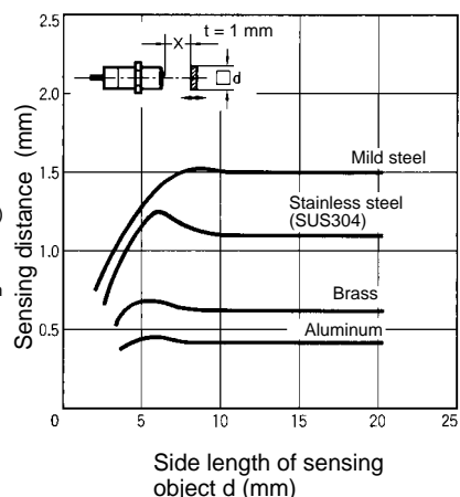
E2E-X1R5E/F E2E-X1R5Y
