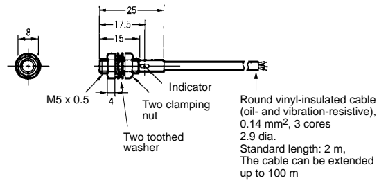
Fig. 2 : E2E-X1□□
