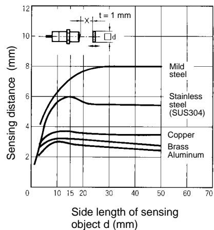
E2E-X1R5E/F E2E-X1R5Y
