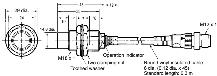
Fig. 32 : E2E-X14MD1-M1GJ
