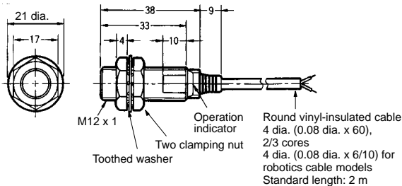
Fig. 8 : E2E-X3D□-N E2E-X2E□/F□
