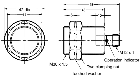
Fig. 25 : E2E-X10D□-M1G/E2E-X10E□-M1/F□-M1 E2E-X10Y1-M1
