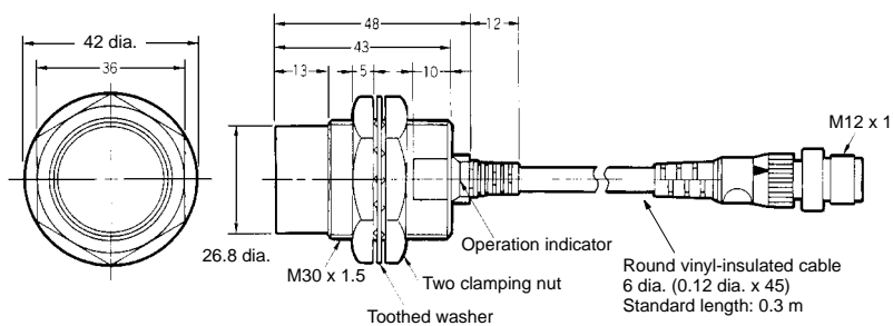
Fig. 34 : E2E-X20MD1-M1GJ
