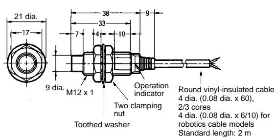
Fig. 9 : E2E-X8MD□ E2E-X5ME□/F□
