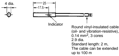
Fig. 3 : E2E-C1□□
