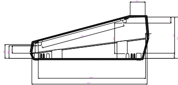
SECCIÓN 1 (DIMENSIONES INTERIORES) SECTION 1 (INNER DIMENSIONS)
