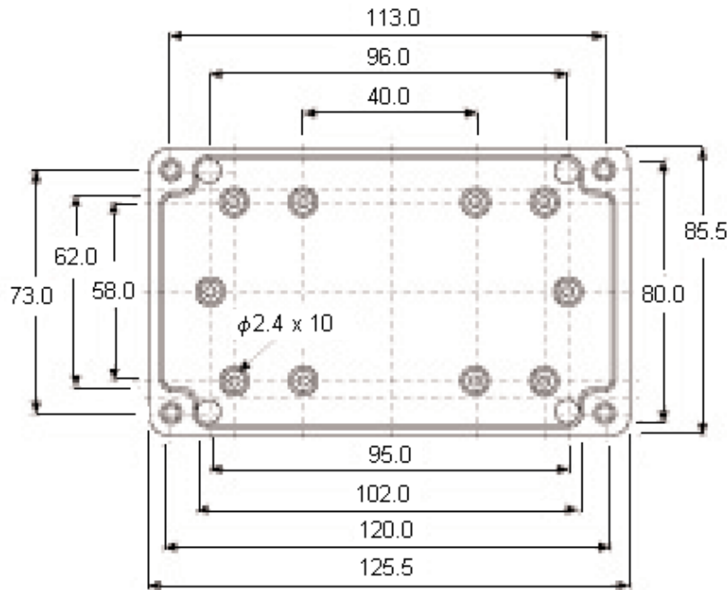
Dimensions : Millimetres
