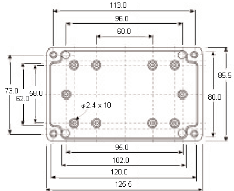
Dimensions : Millimetres
