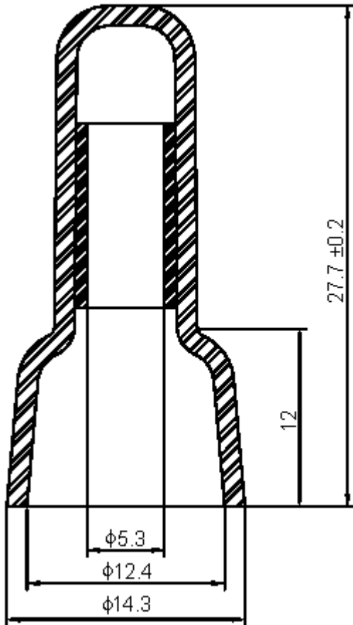
Dimensions : Millimetres
