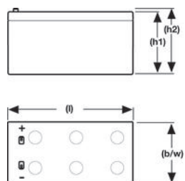
A512/3.5 S
