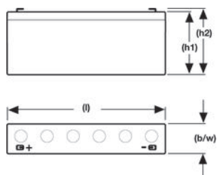
A512/2 S
