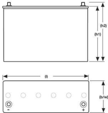
A512/55 A
