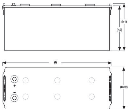
A512/120 A
