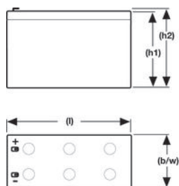
A512/6.5 S
