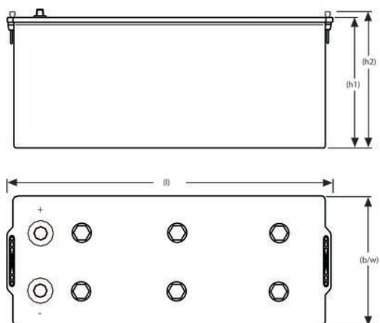
A512/200 A
