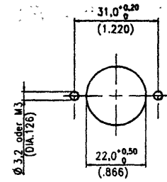
Montageausschnitt / Panel cutout
