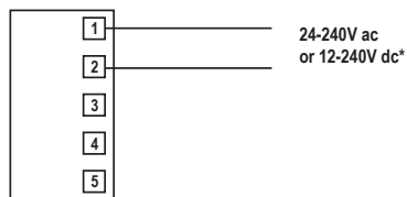
Q853E Emitter
