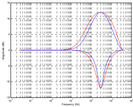
Figure 53 EQ Band 4 – EQ3BW=0, EQ3BW=1
