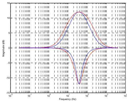
Figure 47 EQ Band 2 – EQ2BW=0, EQ2BW=1
