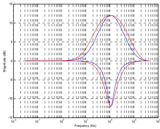
Figure 50 EQ Band 3 – EQ3BW=0, EQ3BW=1
