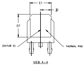
VIEW A-A
