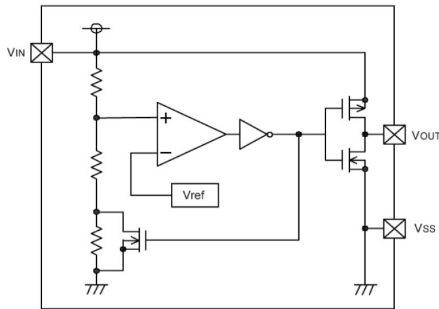
(1) CMOS Output
