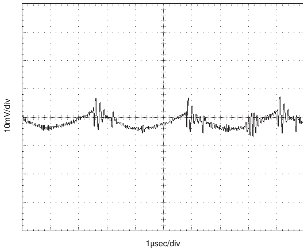
Output Ripple/Noise
