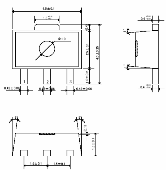
SOT-89
