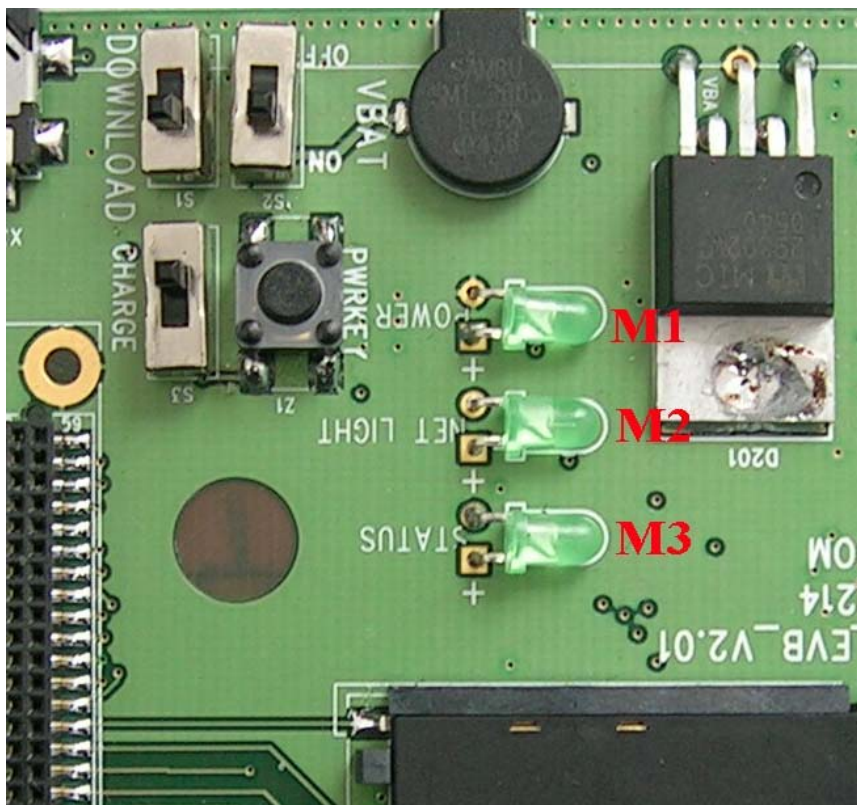
Figure 9: StatusLED
