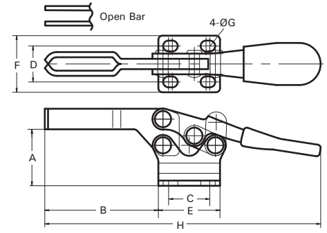
Model GH-201-B Shown
