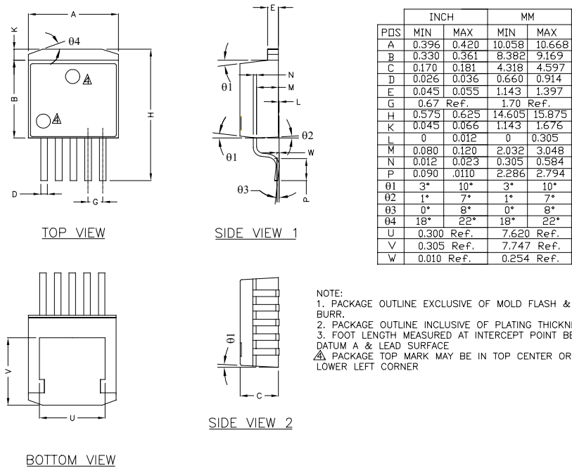
TO-263-5 (U)
