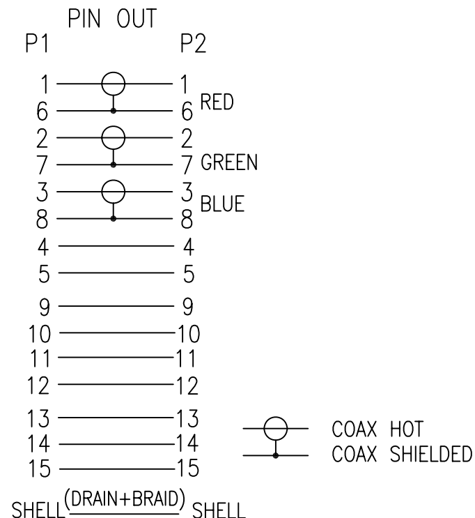
P2 HDB15P M
