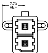
2 CKT
