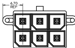
4-12 CKT
