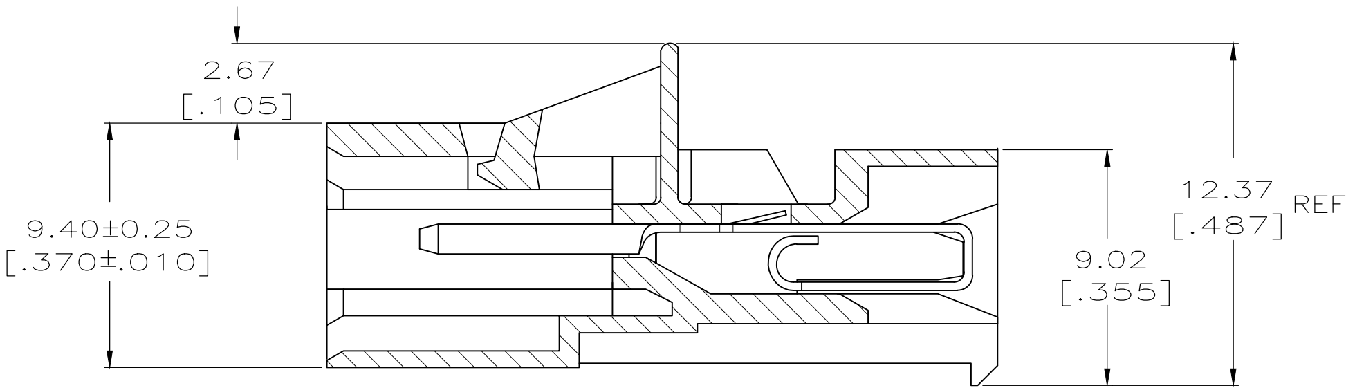
SECTION A-A
