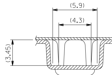
SECT : X-X
