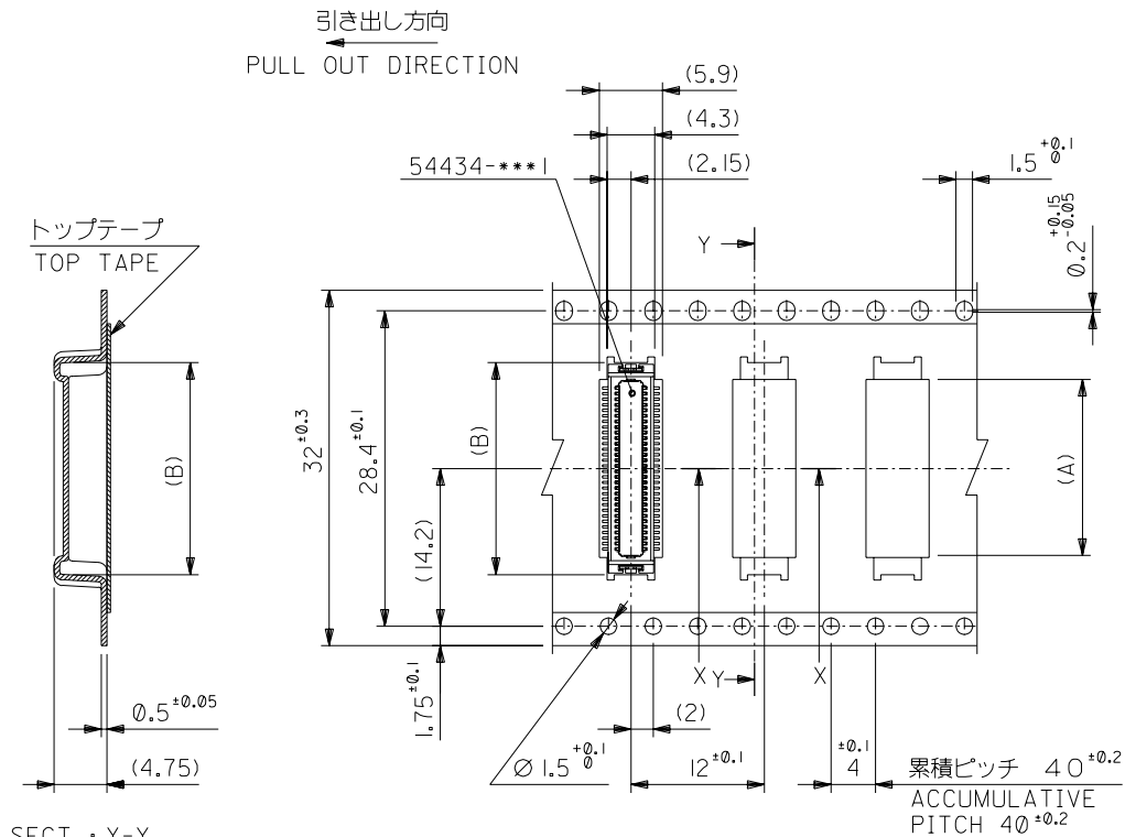
SECT : Y-Y
